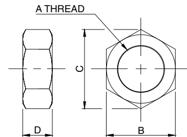
Jam Nut
